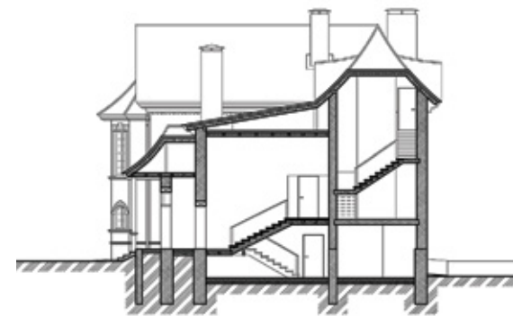
Рис. 3. Разрез дома
